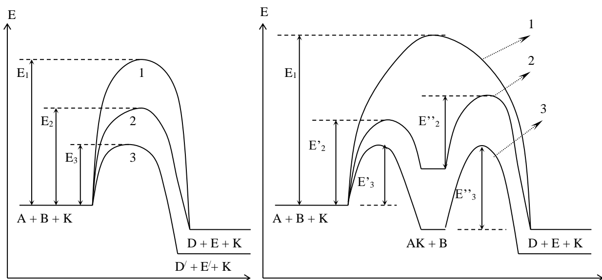
1 - сурет. A+B \rightarrow D+E реакциясының активтену энергиясына катализатордың әсері:
